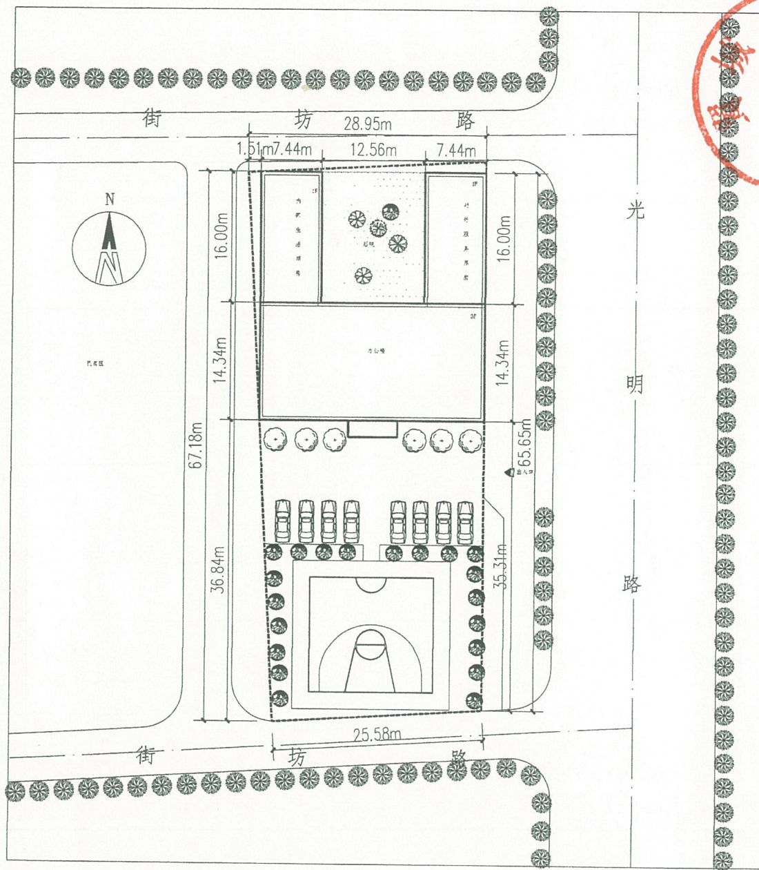
城管派出所总平面图 1:500
