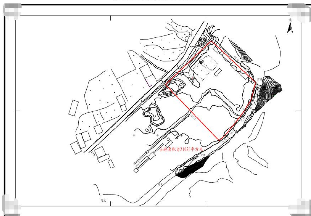
翼城县民兵训练基地建设项目勘测定界图
